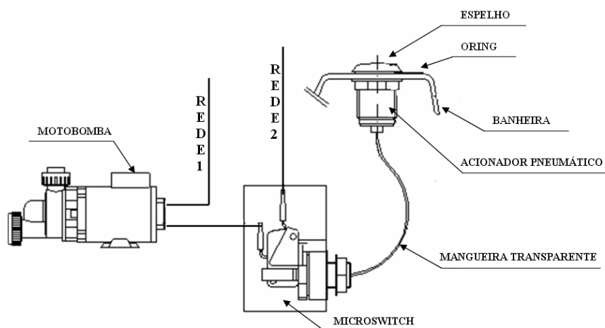
Figura 25 – Motobomba com Acionamento Pneumático
