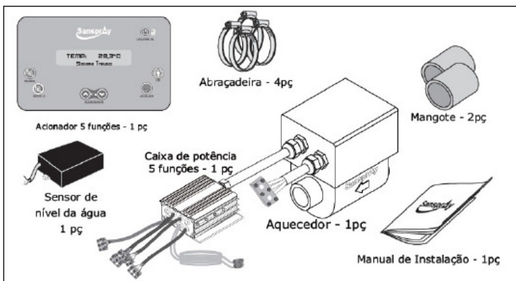
Figura 26 - Componentes do painel controlador 5 Funções
