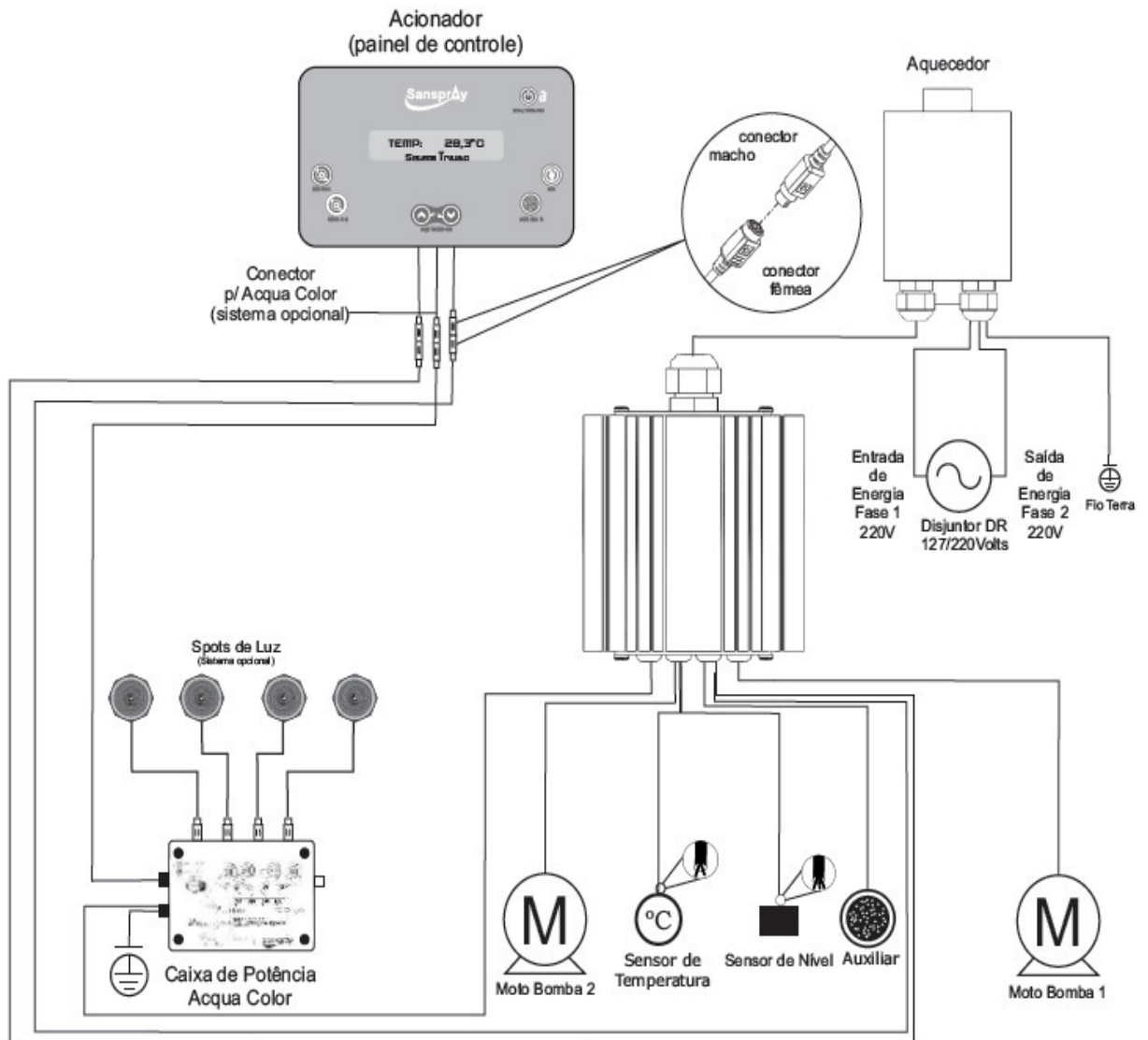
Figura 28 - Diagrama Elétrico do painel controlador 5 Funções
