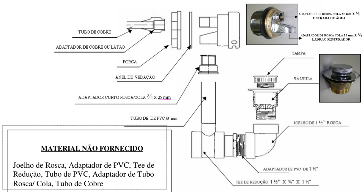
Figura 21 – Ligação Válvula de Escoamento com ladrão misturador
