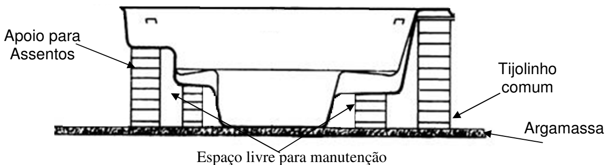
Figura 23 – Assentamento em alvenaria
