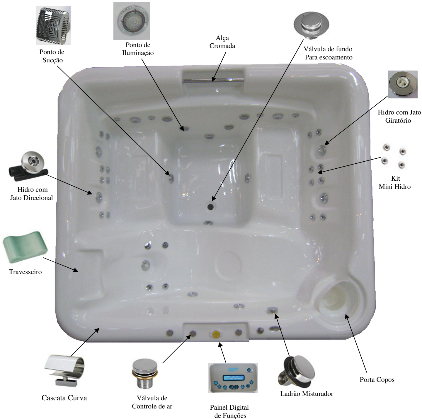
Figura 2 – Configuração Externa
