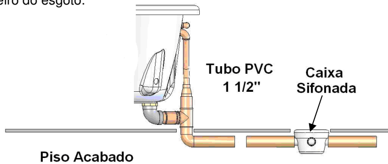
Figura 22 - Válvula de Saída ao Ponto de Esgoto
