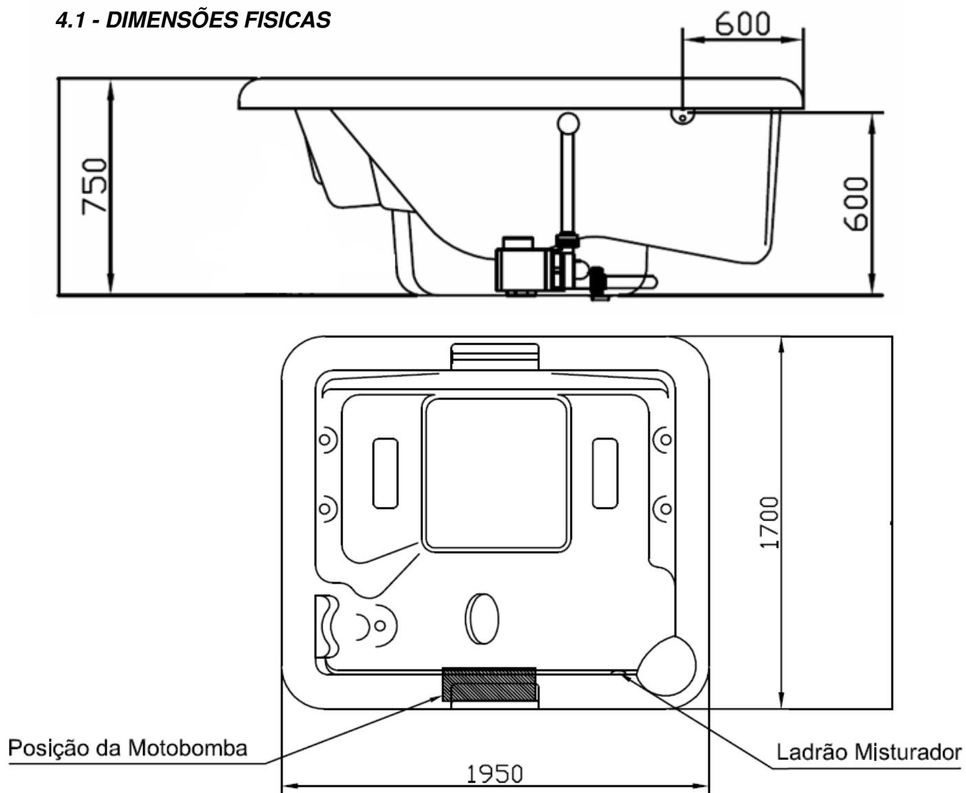
Figura 1 – Dimensões Físicas Externas
