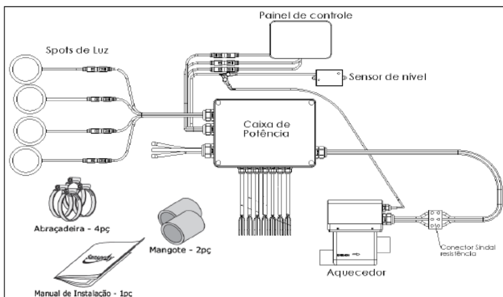
Figura 27 - Componentes do painel 8 Funções
